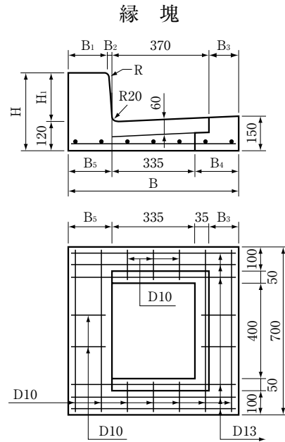
国土交通省L形縁塊 (単位 m/m)
