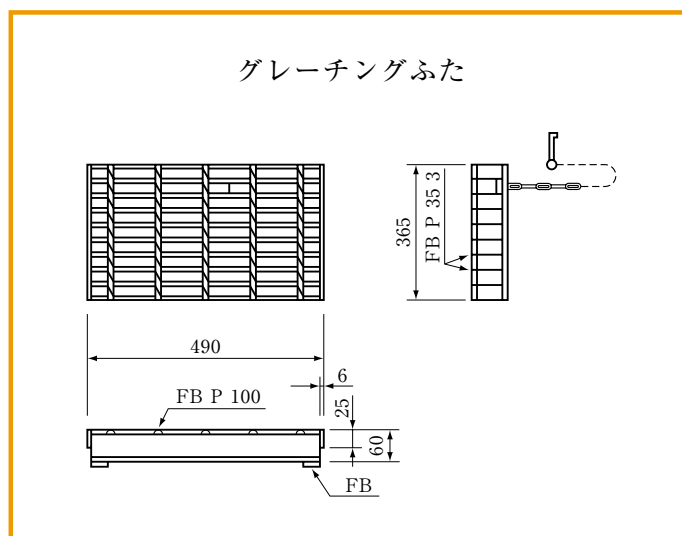
国土交通省L形縁塊ふた(グレーチング)
