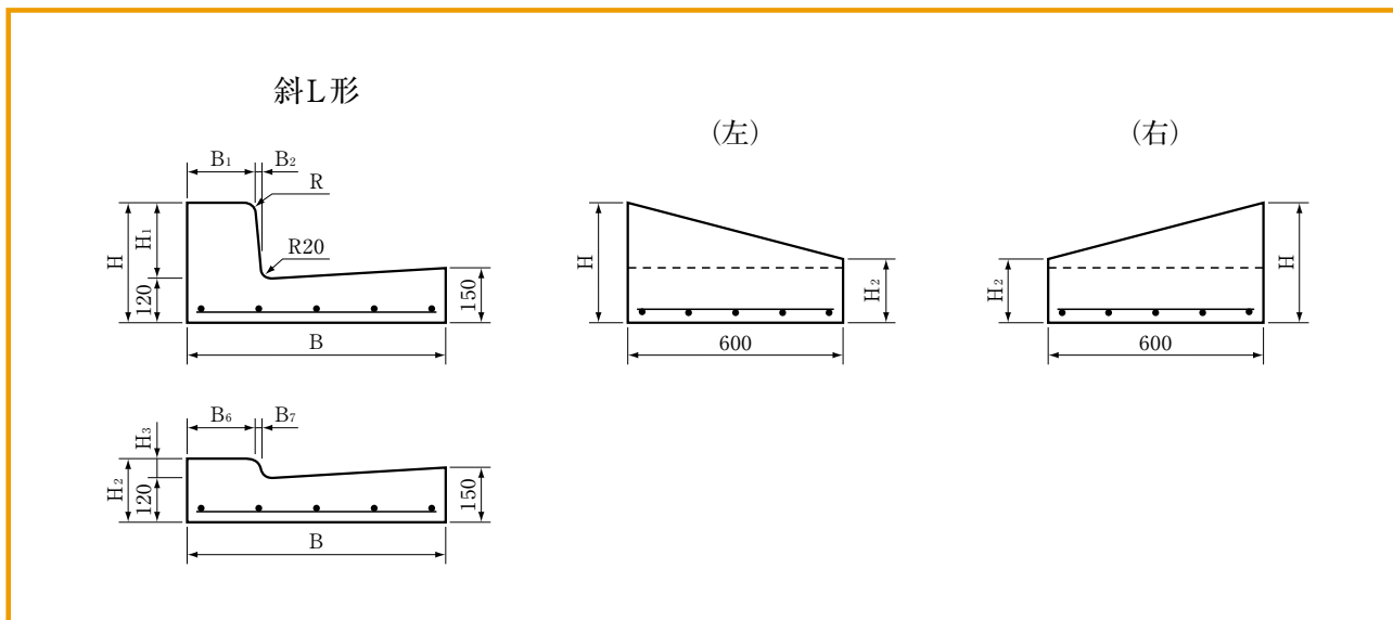
国土交通省L形
