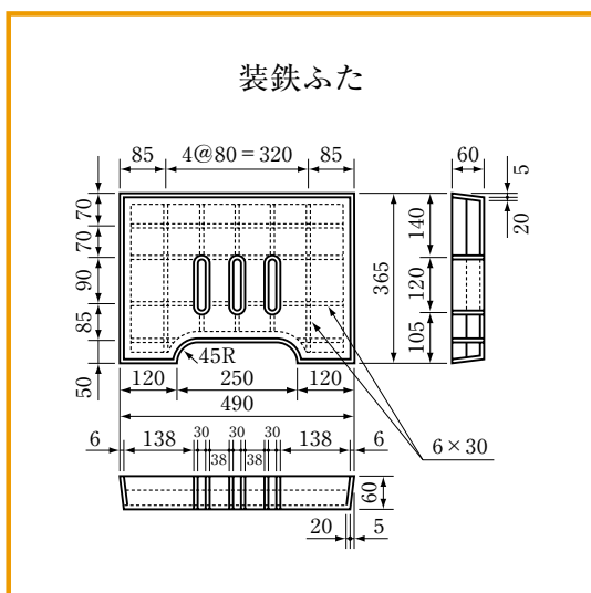
国土交通省L形縁塊ふた
