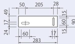
プレキャスト街きよ用連結プレート 90×283×4.5mm
