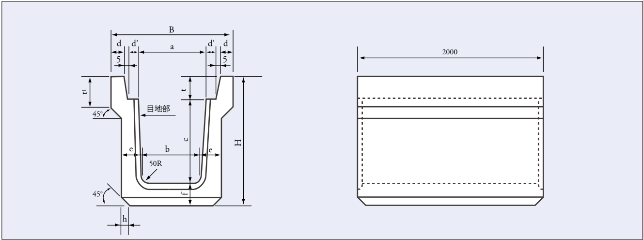
目地部詳細図 1種・3種 単位mm
