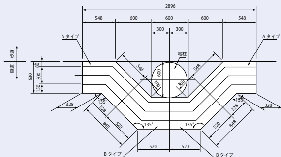
電柱切り廻し部
