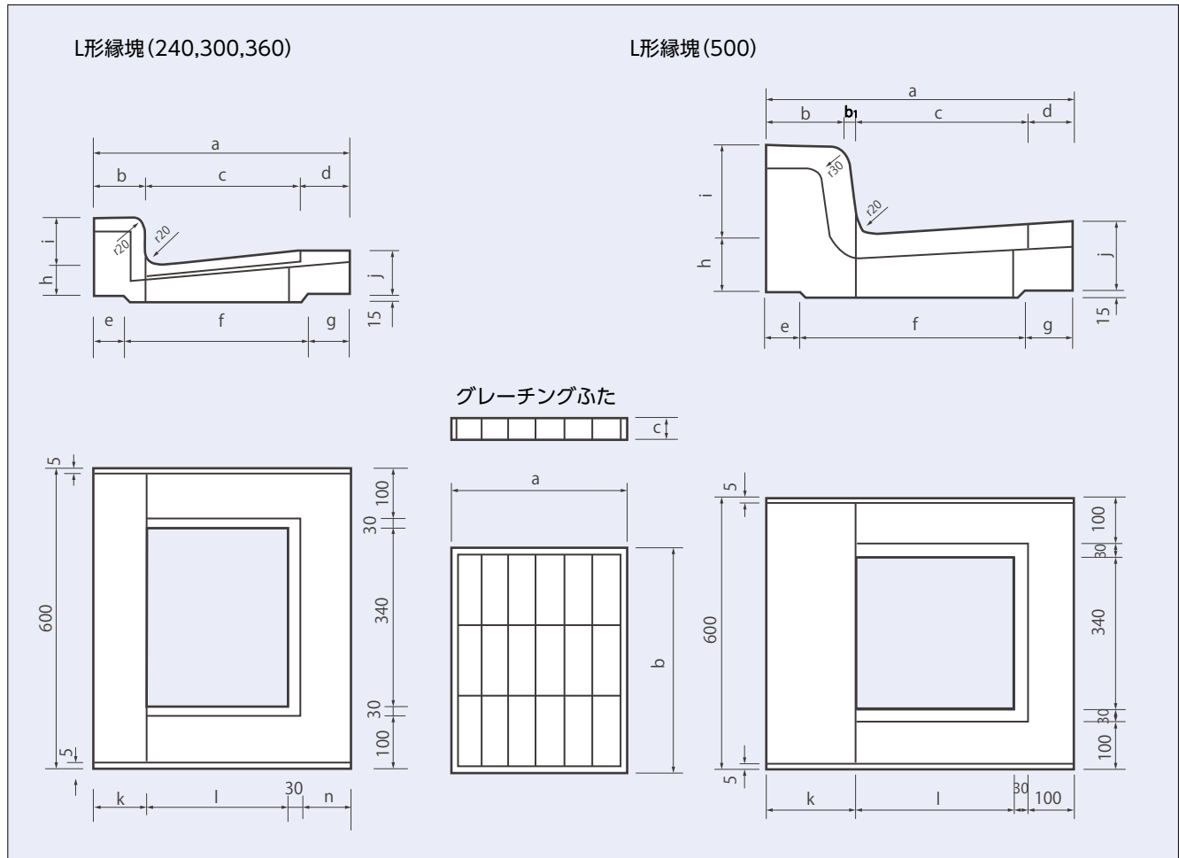
L形縁塊寸法表
