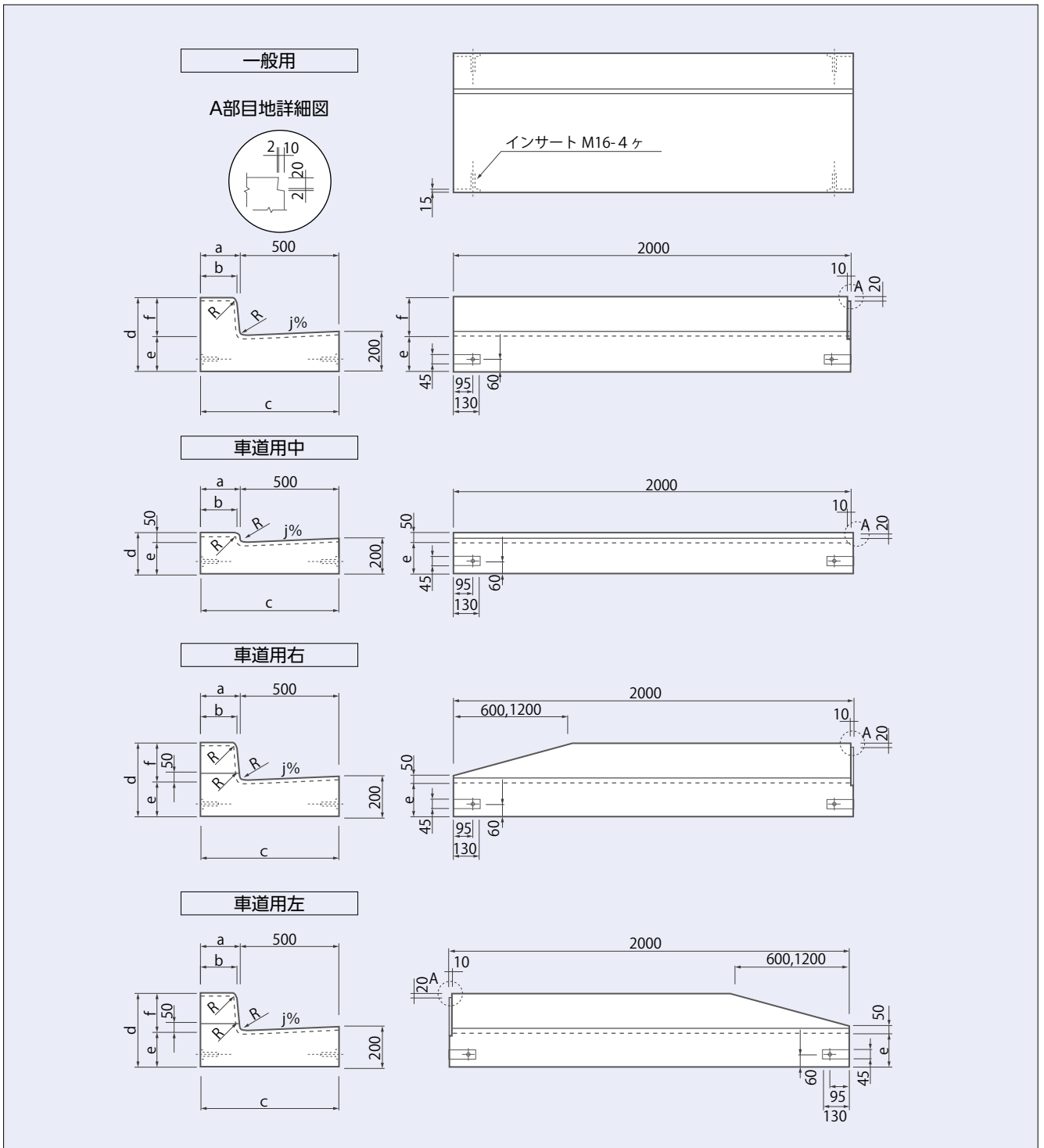
プレキャスト街きょ205型
