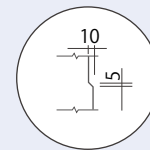
A部目地詳細図
