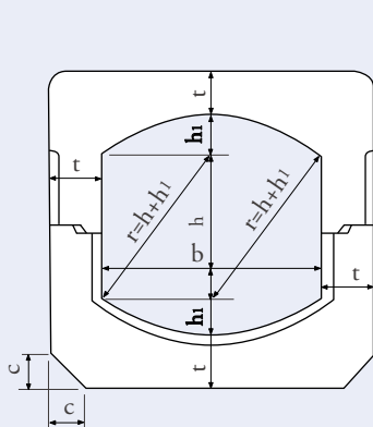
断面
