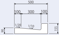
標準 600×500×155 質量65kg
