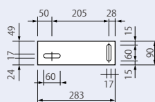
プレキャスト街きよ用・縁塊連結プレート 90×283×4.5mm
