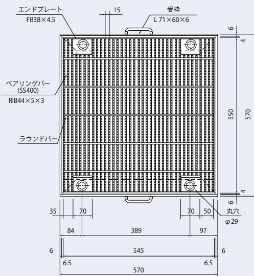
グレーチング細目タイプ
