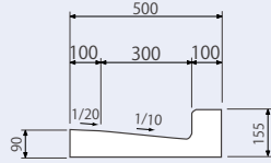
2点段差斜 600×500×155/90 質量61kg
