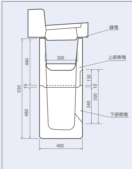
組立図
