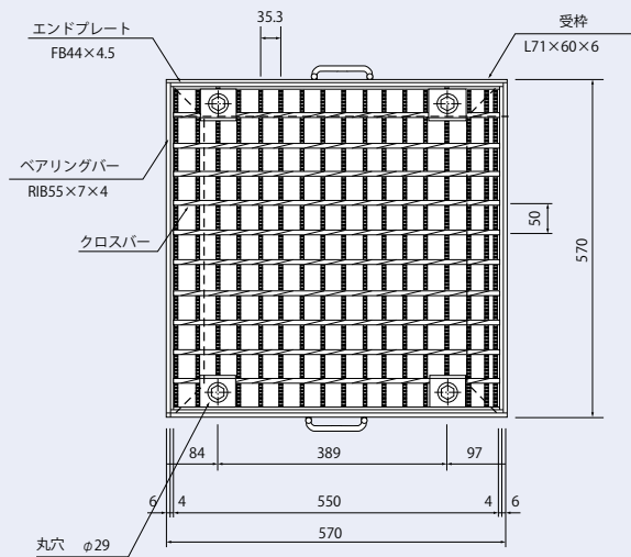
グレーチング標準タイプ
