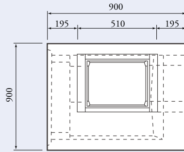
中央断面図
