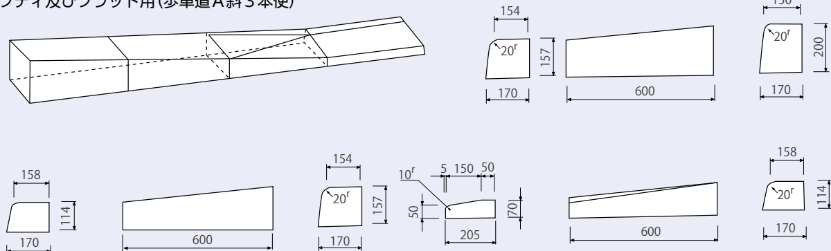
セーフティ及びフラット用(歩車道A斜3本使)
