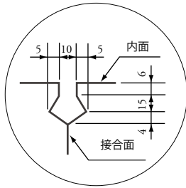
目地部詳細図 1種・3種 単位mm
