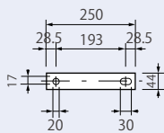
プレキャスト街きよ用連結プレート 40×250×4.5mm
