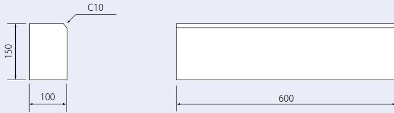
100×150×600
