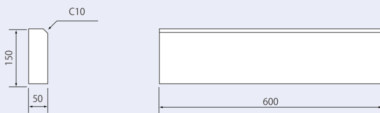
50×150×600 (半コーピンタイプ)
