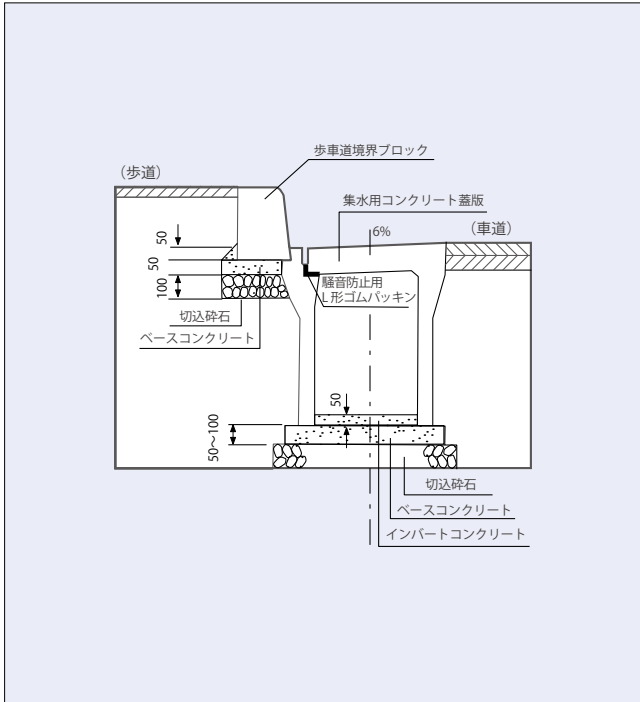
標準断面
