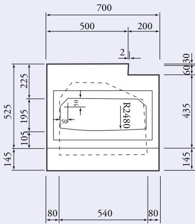
BOX 側正面図
