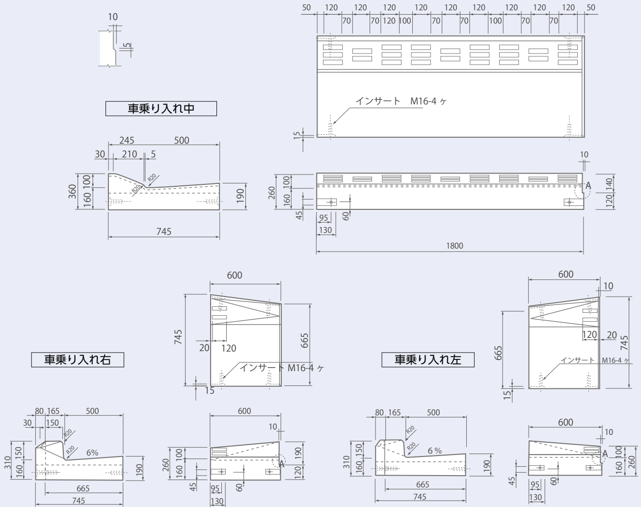
プレキャスト街きょ155- I
