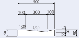
2点段差平 600×500×90 質量58kg
