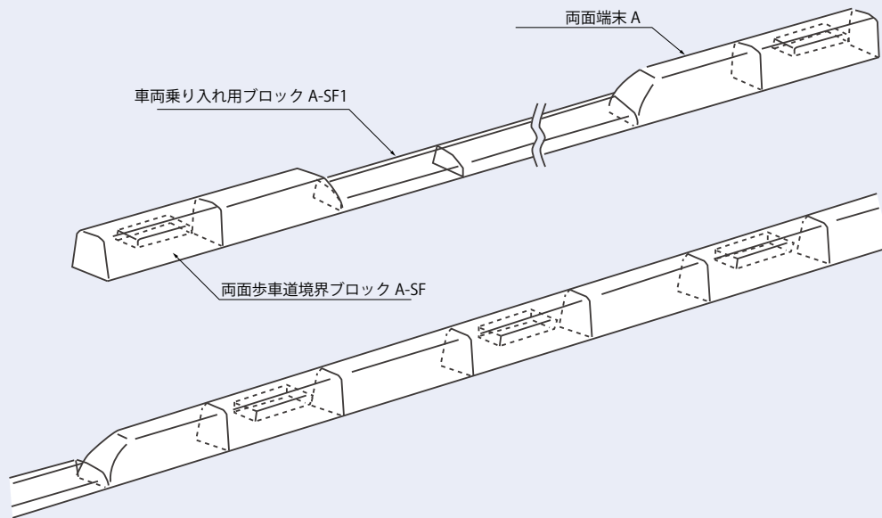
施工図
