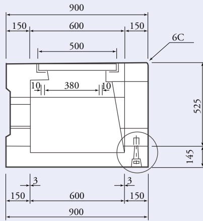
中央断面図
