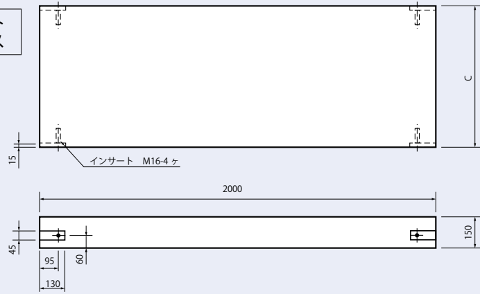
プレキャスト街きよベース
