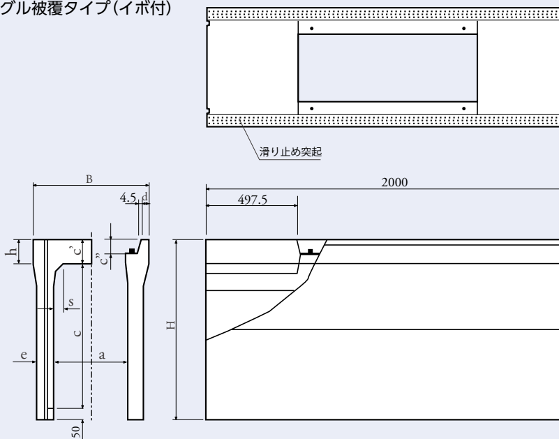
●VS側溝[横断用]アングル被覆タイプ(イボ付)
