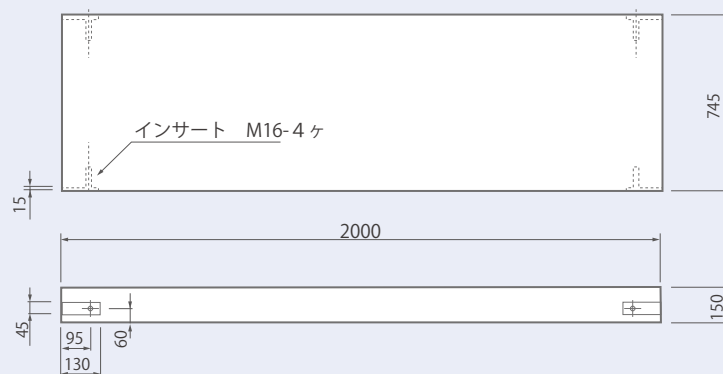
プレキャスト街きょ用ベース
