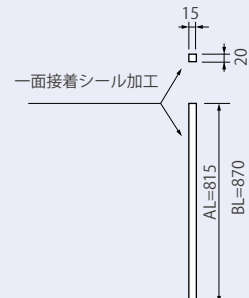
プレキャスト街きよ用目地材 (材質:ポリウレタン系)
