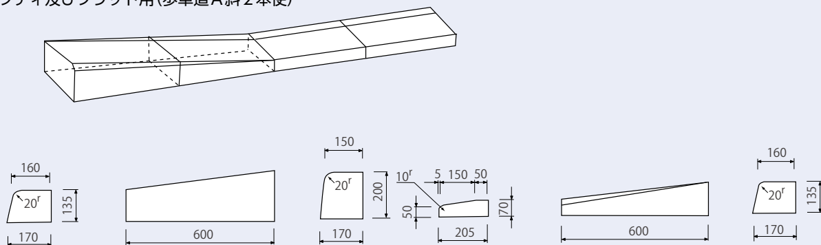
セーフティ及びフラット用(歩車道A斜2本使)
