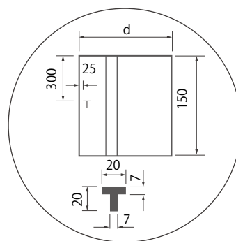
Tマーク詳細図
