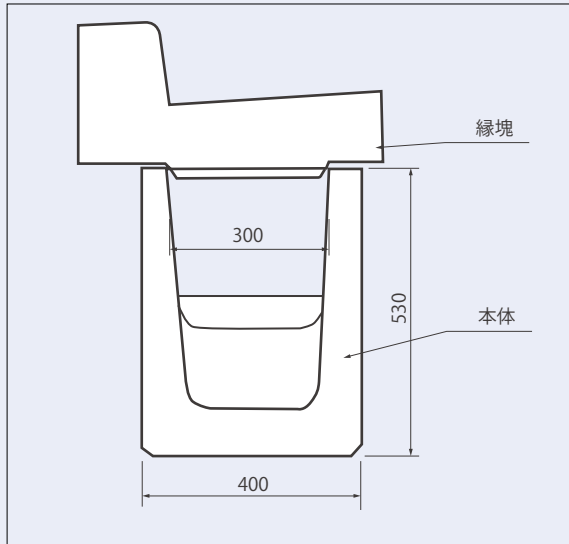
組立図
