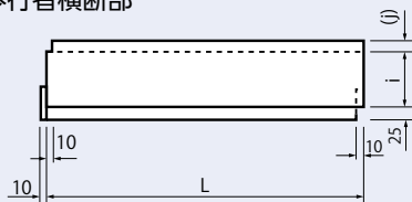
歩行者横断面部
