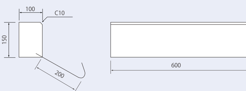
100×150×600 (鉄筋出し)
