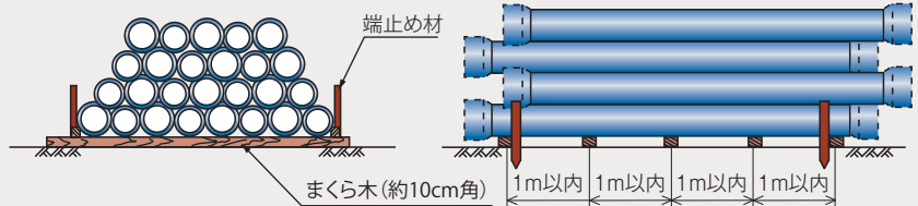
目積み(千鳥積み)する場合(1本梱包)
